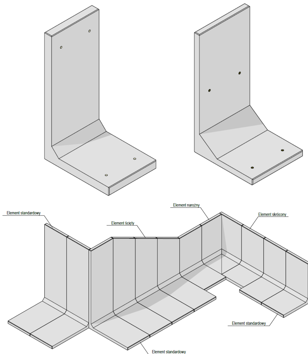
Rysunek 4.2-3: Sienkiewicz MAT-BUD Sp. z o. o. – wizualizacja elementów ścian oporowych
